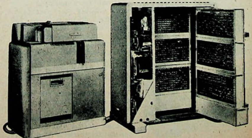
Een spectaculair „nieuwtype” op de Jaarbeurs was deze elektronische rekenmachine. De beide rekken zijn gevuld met 1200 buizen...
